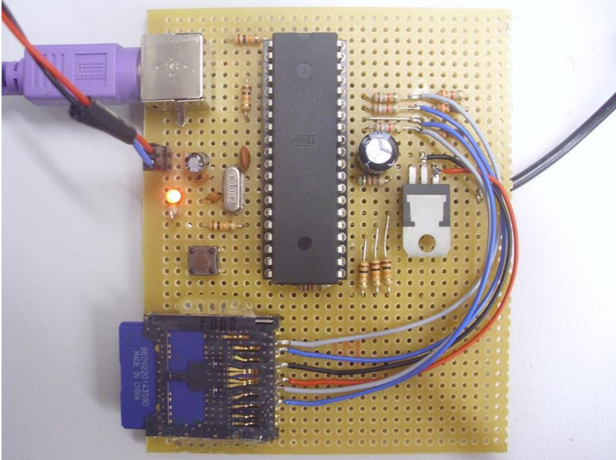
Lochrasteraufbau:
