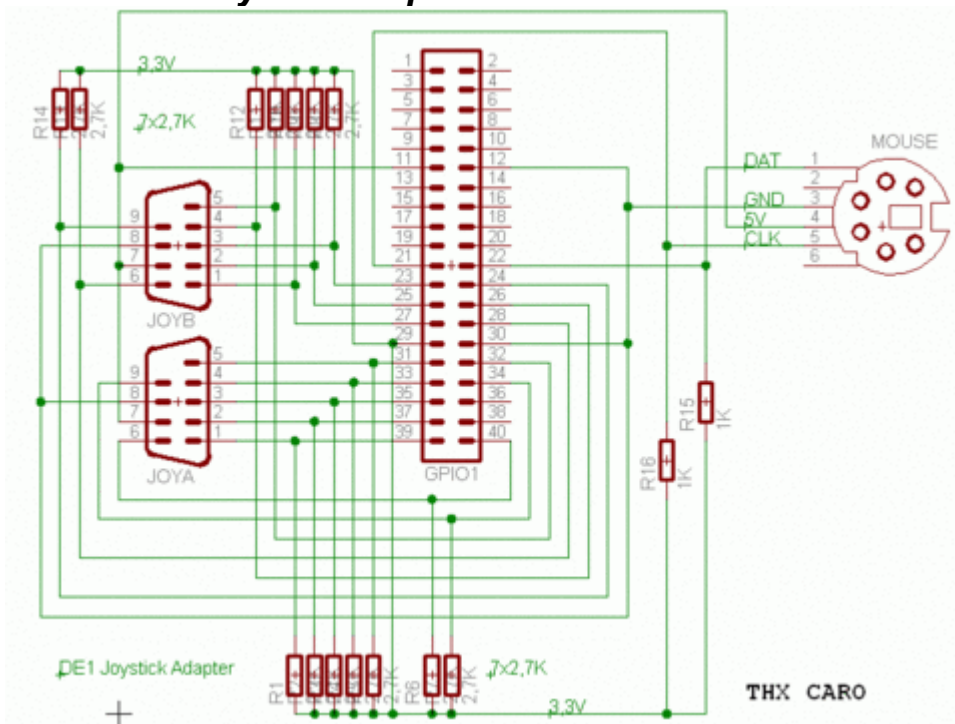
Schaltbild Joystickadapter
