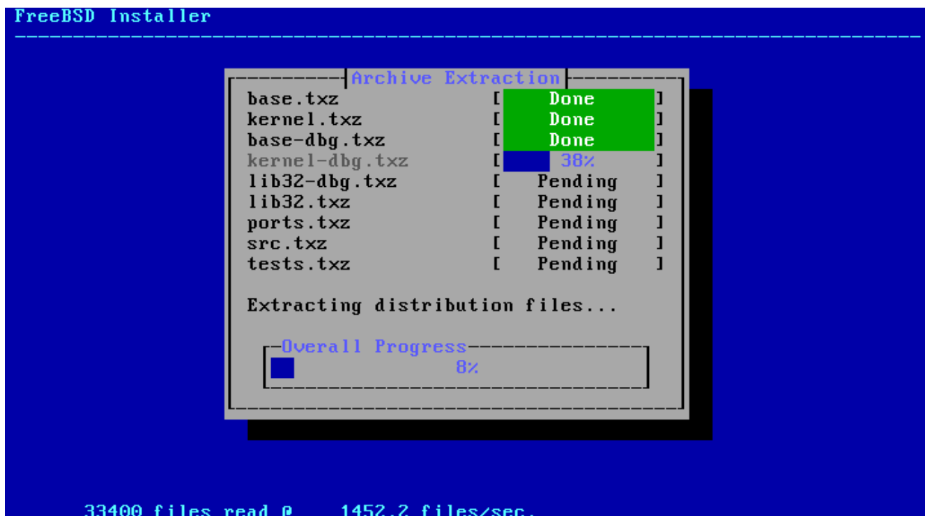
Рисунок 33. Извлечение файлов дистрибутива
