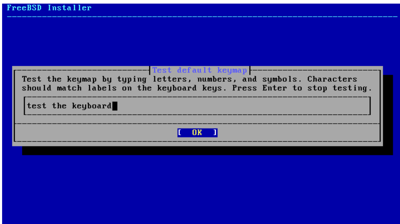
Рисунок 6. Меню тестирования раскладки клавиатуры
