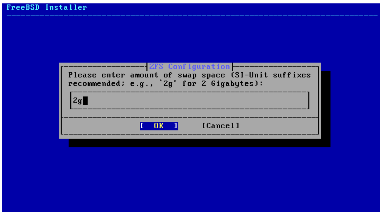
Рисунок 27. Размер раздела подкачки
