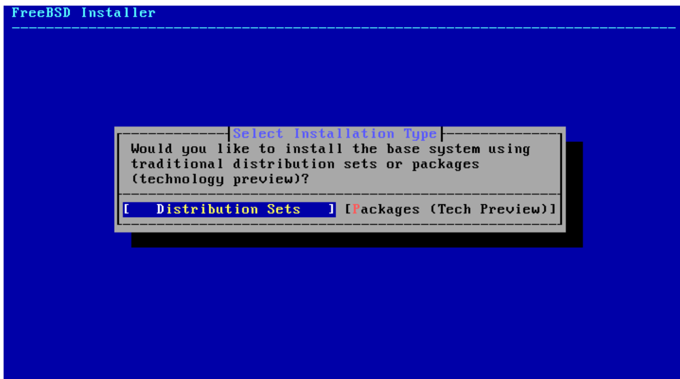
Рисунок 8. Выбор типа установки
