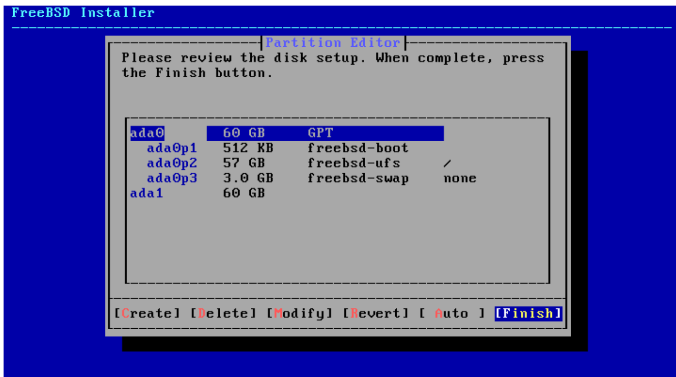
Рисунок 15. Проверка созданных разделов
