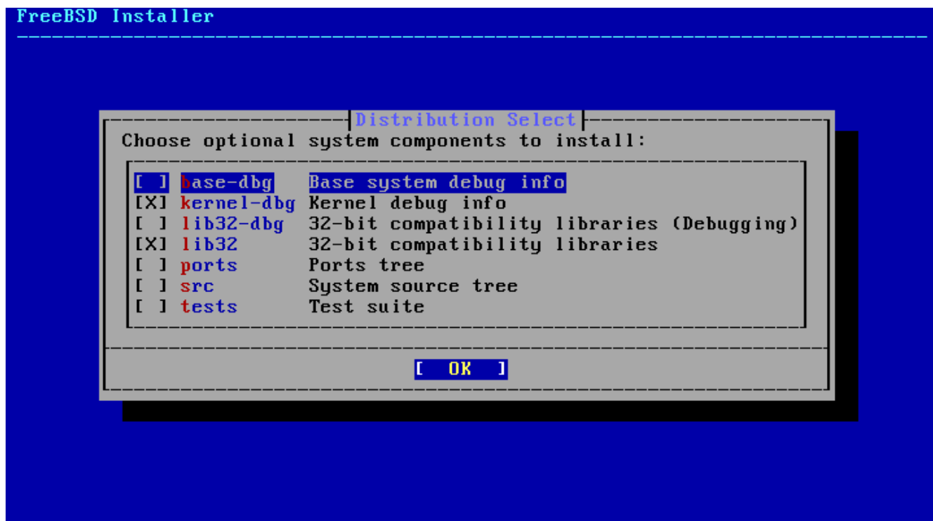
Рисунок 9. Выбор компонентов для установки
