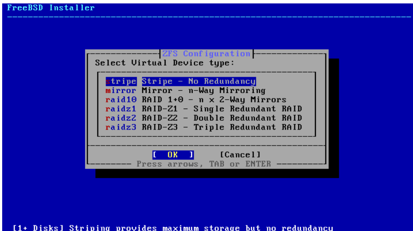
Рисунок 21. Тип пула ZFS
