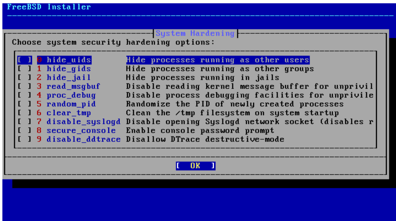
Рисунок 54. Выбор параметров усиленной безопасности
