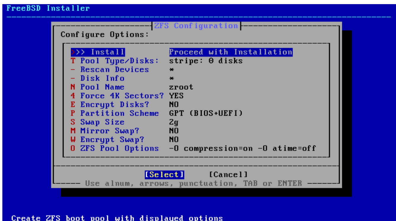
Рисунок 20. Меню разметки ZFS
