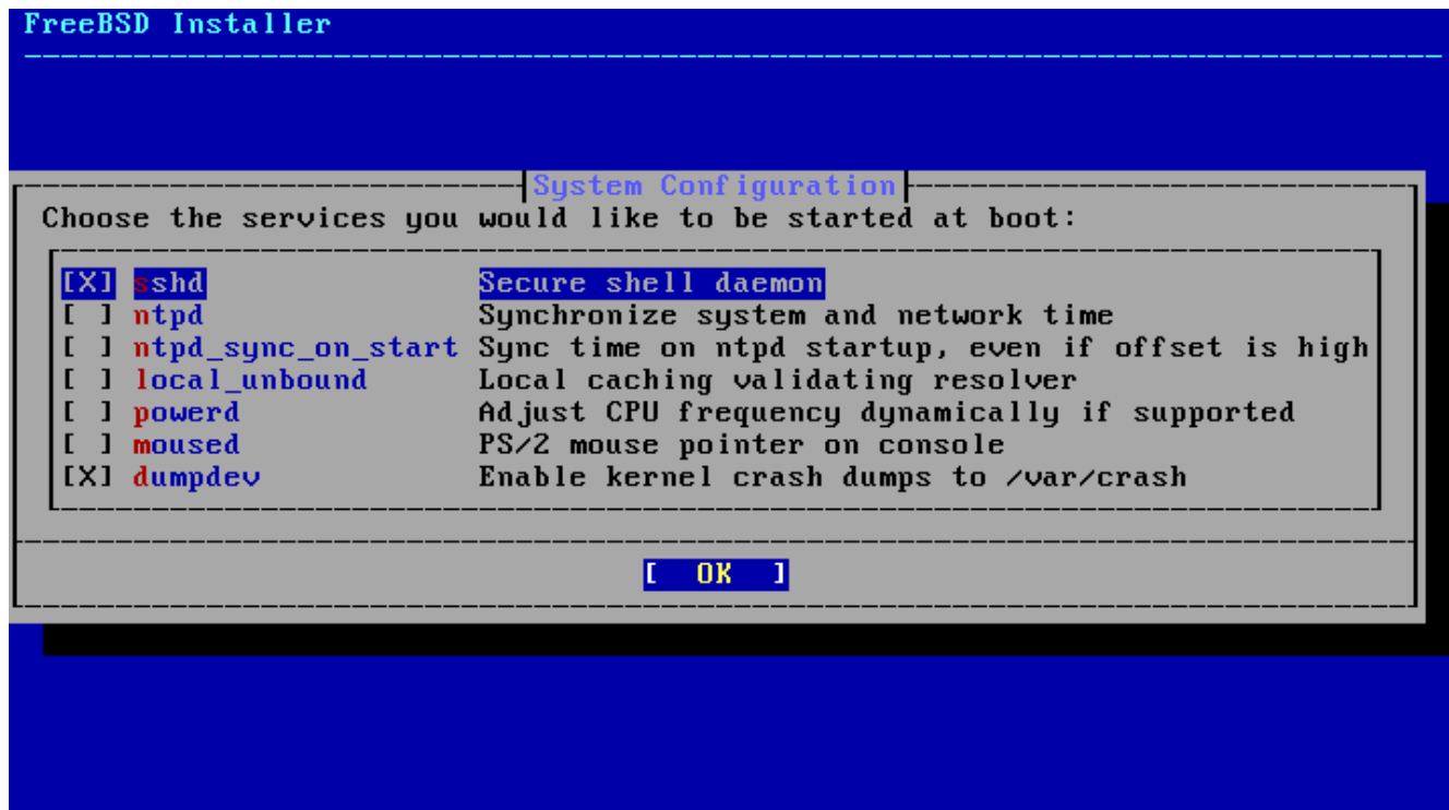
Рисунок 53. Выбор дополнительных служб для включения
